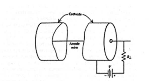
D、G-M 计数管
